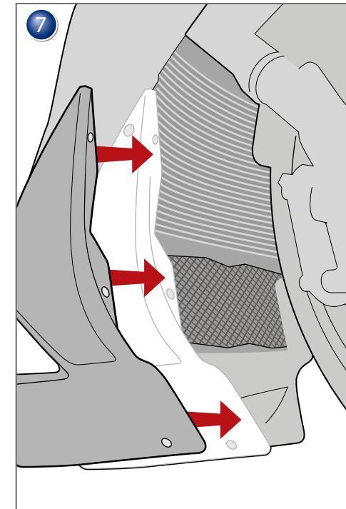
Protección del radiador del aceite Pieza 31961-002
